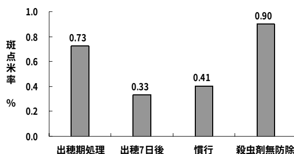
図2 水面施用剤(ジノテフラン粒剤)処理と斑点米率 (H16 旭川、ほしのゆめ)
