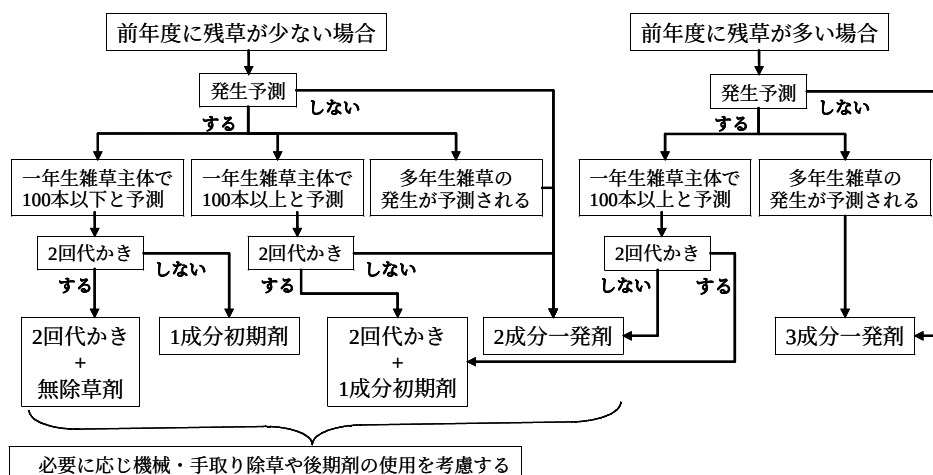
図1 YES!clean 栽培の高度化に向けた雑草防除対応フロー
