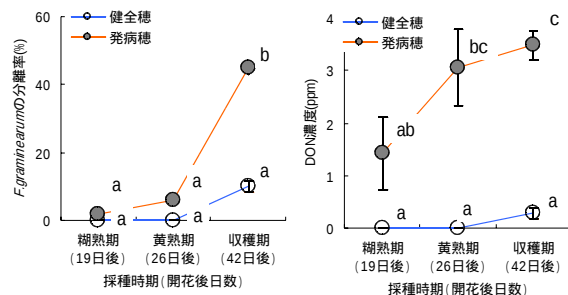
図1 外観健全粒のDON濃度と F. g. の分離率(H17年)
