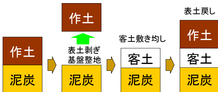
砂質客土埋設工法の施工方法
