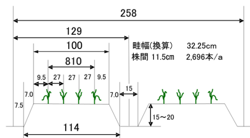
図 高畦移植栽培の断面図(単位:cm)
