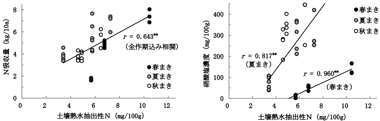
図1. 無N栽培条件における土壌熱抽NとみずなN吸収量（左）・硝酸塩濃度（右）との関係
