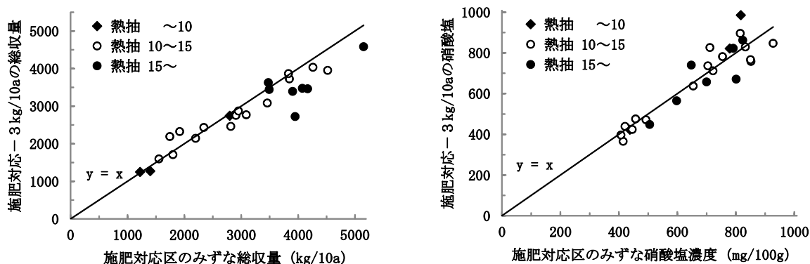
図2. 土壌熱抽N水準別にみた窒素施肥量「施肥対応」と同「施肥対応マイナス3 kg/10a」との関係
