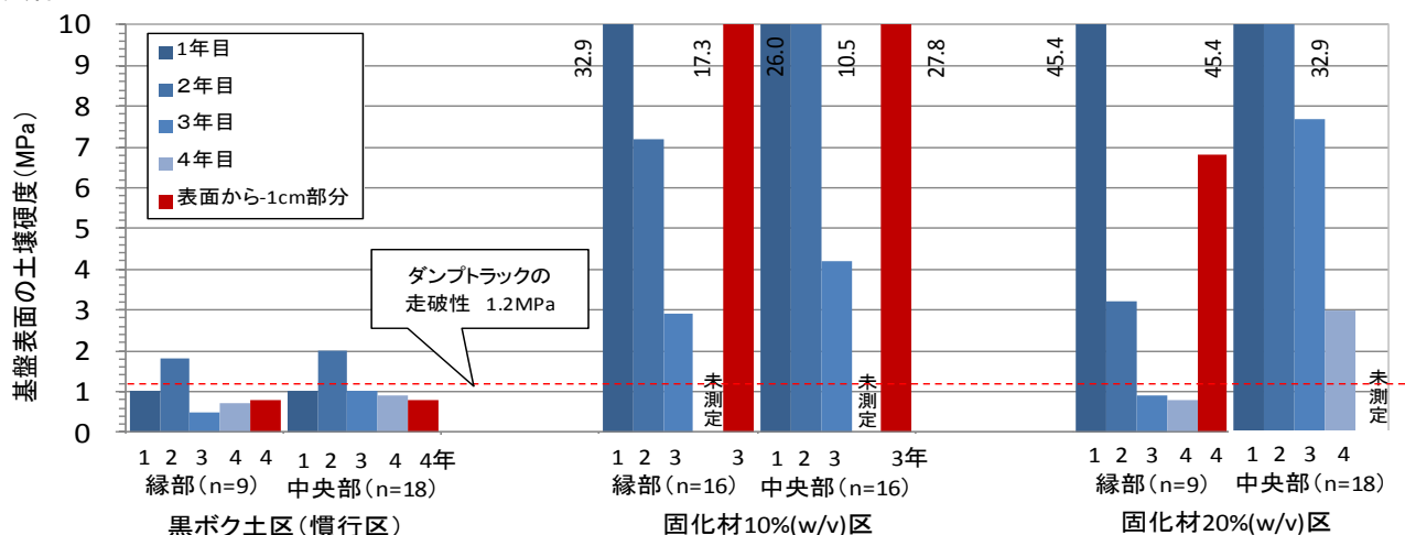
図1 セメント系固化材混合基盤の土壌硬度（山中式硬度計を基盤表面に対し垂直貫入による計測）の経年変化
