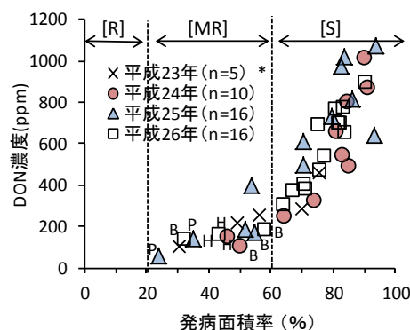
図 1 有傷接種法における早生品種の赤かび病発病面積率と DON 濃度の関係 データラベルは品種記号 (表 1 と共通), *括弧内の数字は供試品種数, 発病面積率 0～20%: [R] (抵抗性), 21～60%: [MR] (中程度抵抗性), 61%以上: [S] (感受性)
