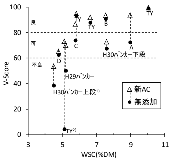
図1 原料草のWSC含量とサイレージV-Scoreの関係
