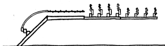
図2 片側水平コルドン(更新式)
