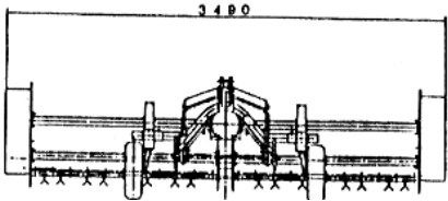
図1 4畦用茎葉チョップパ概略図
