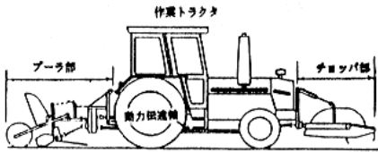
図2 馬鈴しょ茎葉引き抜き機の概略図
