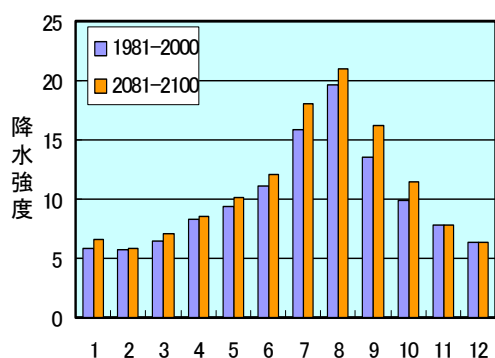
図10 北日本日本海側の降水強度（降水量／降水日数）の変化
