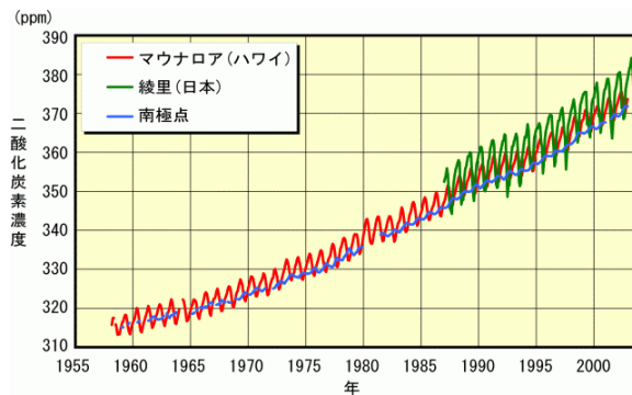
図5 大気中の二酸化炭素濃度の上昇
