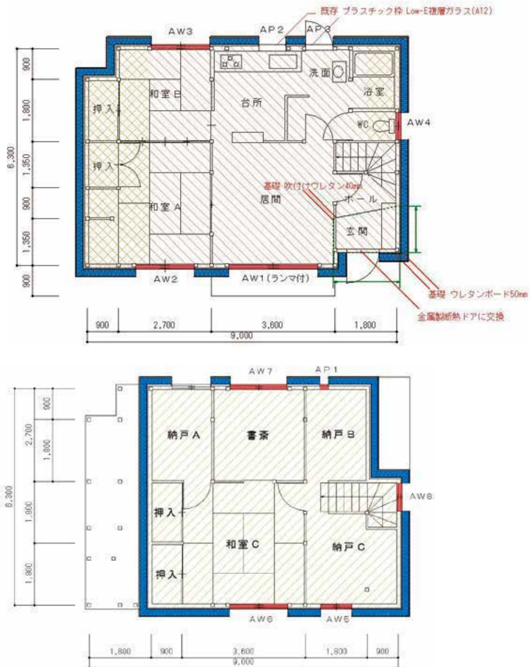
図2 平面図（改修後）
