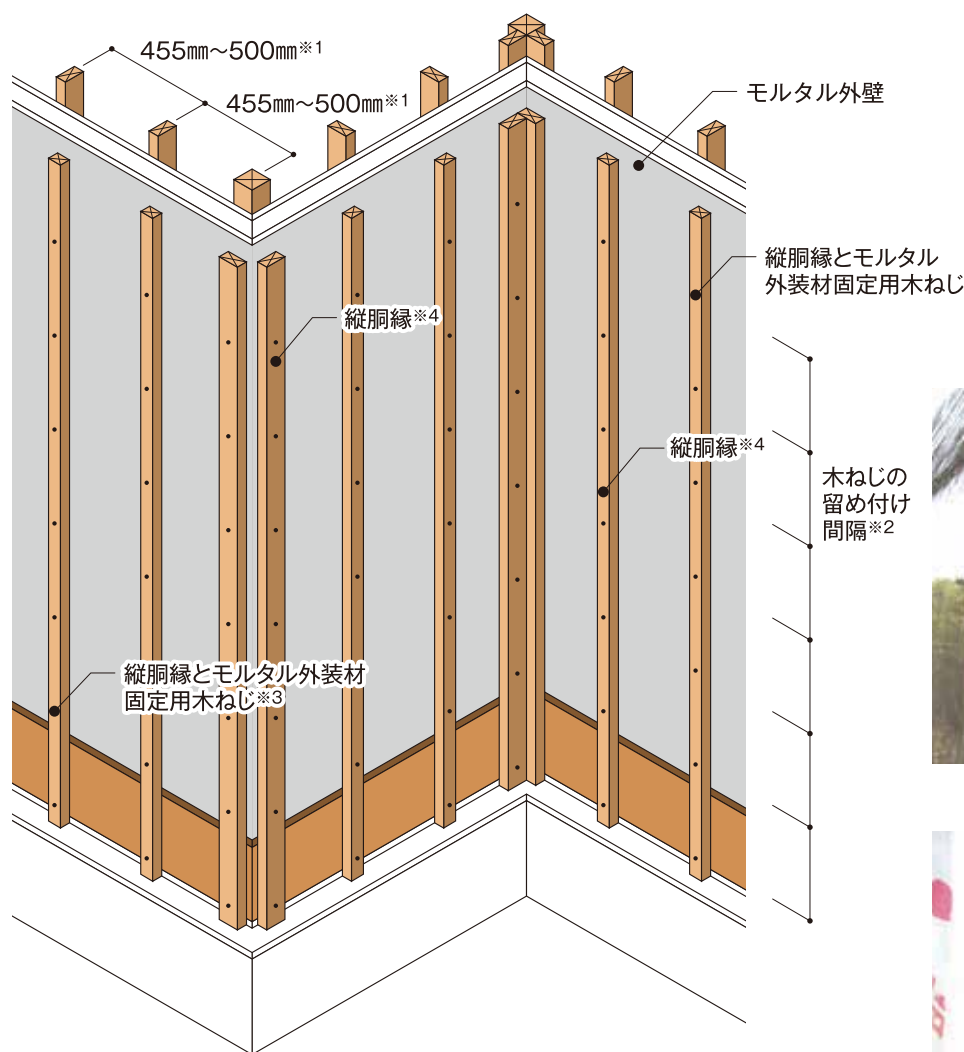
パネリードP6×120Ⅱ+ (東日本パワーファスニング(株)製)
