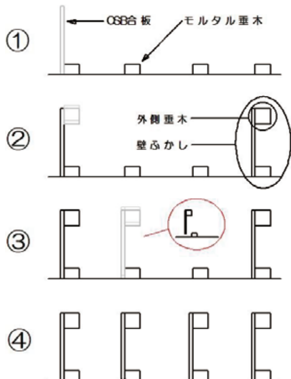
図5 壁ふかし施工手順
