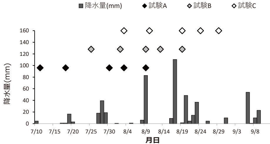
図2 2016年中央農試の薬剤散布試験における散布月日と降水量
