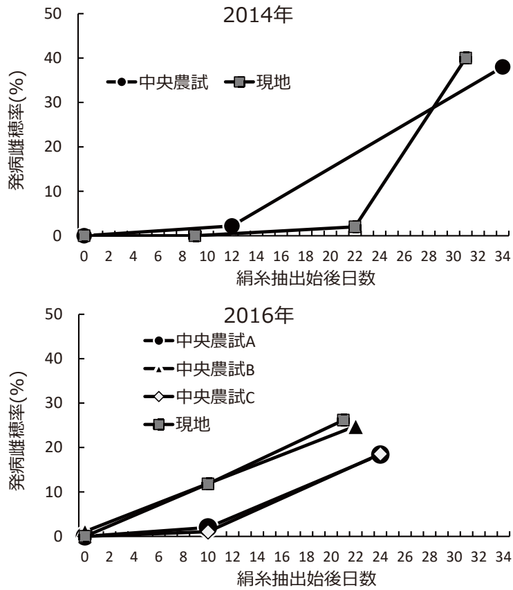
図1 無防除区における絹糸抽出後日数と発病雌穂率の推移
