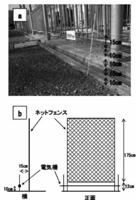
図4 キツネ対策事例 a:電気柵設置（10～15cmで4～5段） b:物理柵との組み合わせ事例（下段1段のみ電気柵設置）
