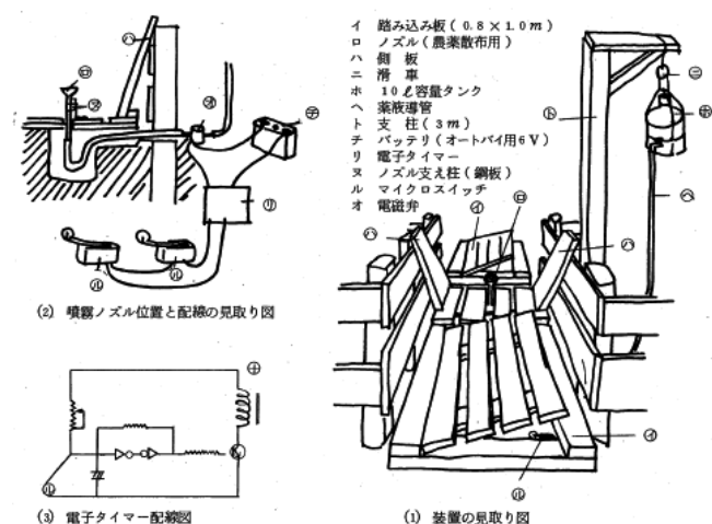
図1 下腹部散布器具の見取り図と配線図
