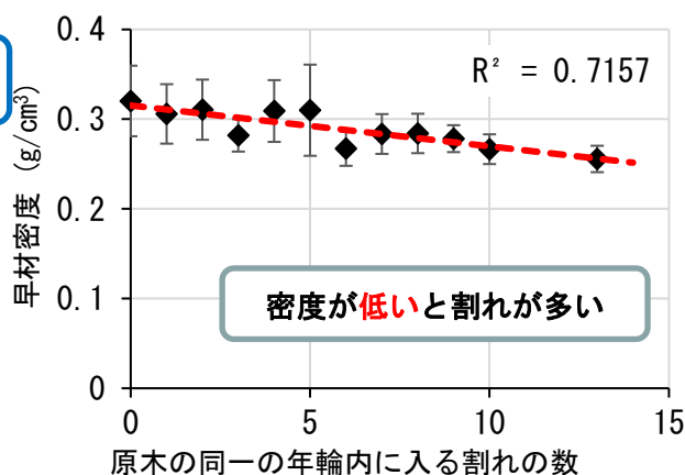
図3 同一の年輪内に発生する割れの数と早材密度（1年輪割れのデータのみ）
