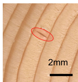
写真1 1年輪割れ
